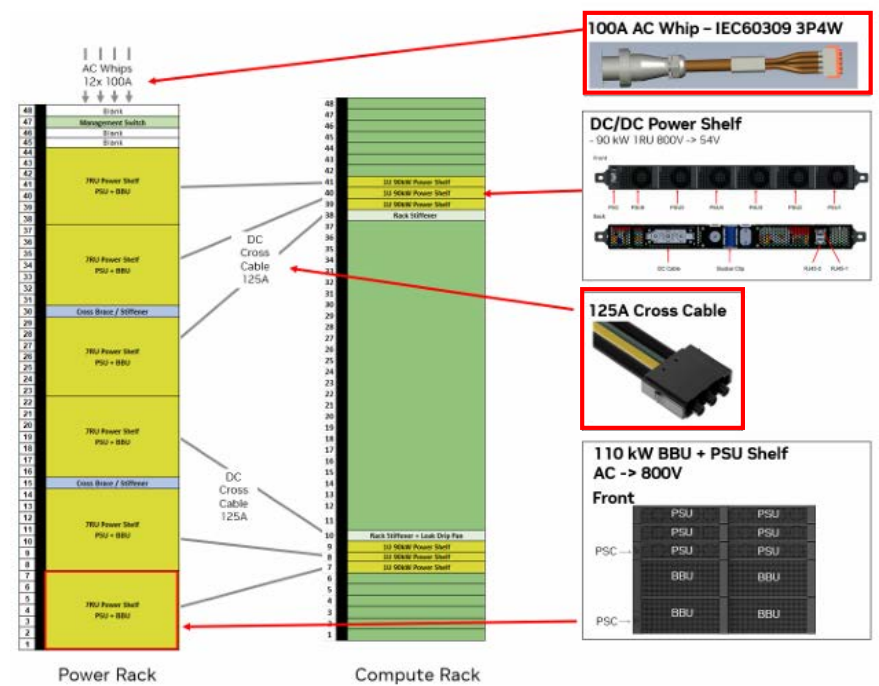
圖 9：Nvidia (美) 800V DC 第一代電源櫃參考設計
