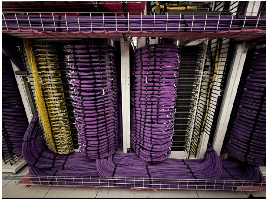
圖 8：用於 xAI (美) 伺服器機櫃之 AEC (紫)
